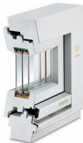
HF 90
