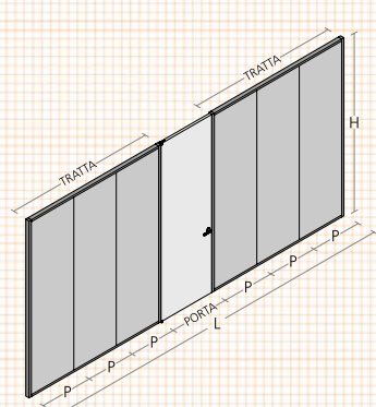
codice code SWPLSW Anta battente / Swing door
