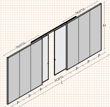
codice code SWPLSL Anta scorrevole / Sliding door
