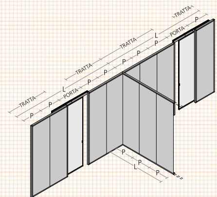
codice code SWPS3VSL Anta scorrevole / Sliding door
