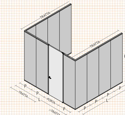
codice code SWPSW Anta battente / Swing door
