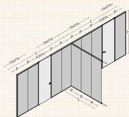
codice code SWPS3VSW Anta battente / Swing door
