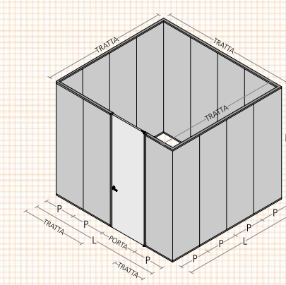
codice code SWISW Anta battente / Swing door
