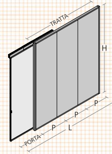
codice code SWPLSL Anta scorrevole / Sliding door
