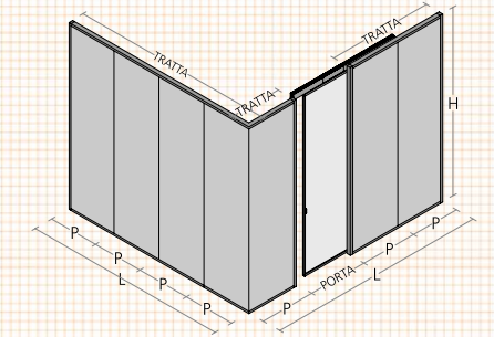
codice code SWPASL Anta scorrevole / Sliding door
