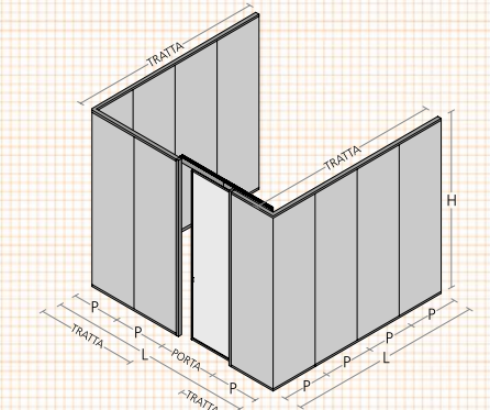
codice code SWPSL Anta scorrevole / Sliding door
