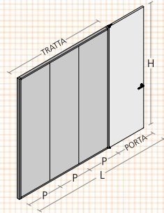
codice code SWPLSW Anta battente / Swing door
